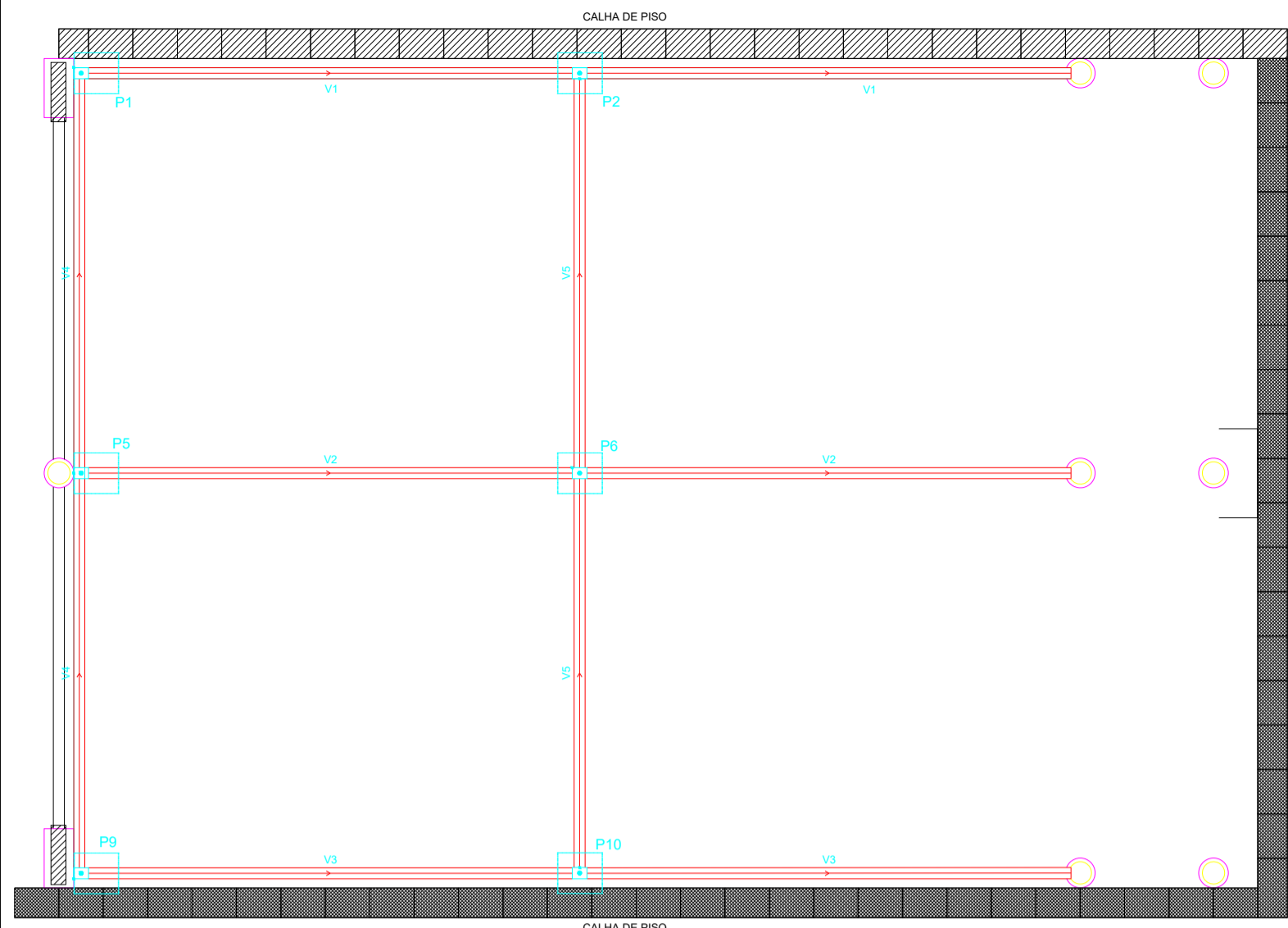
Vigas Baldrame
