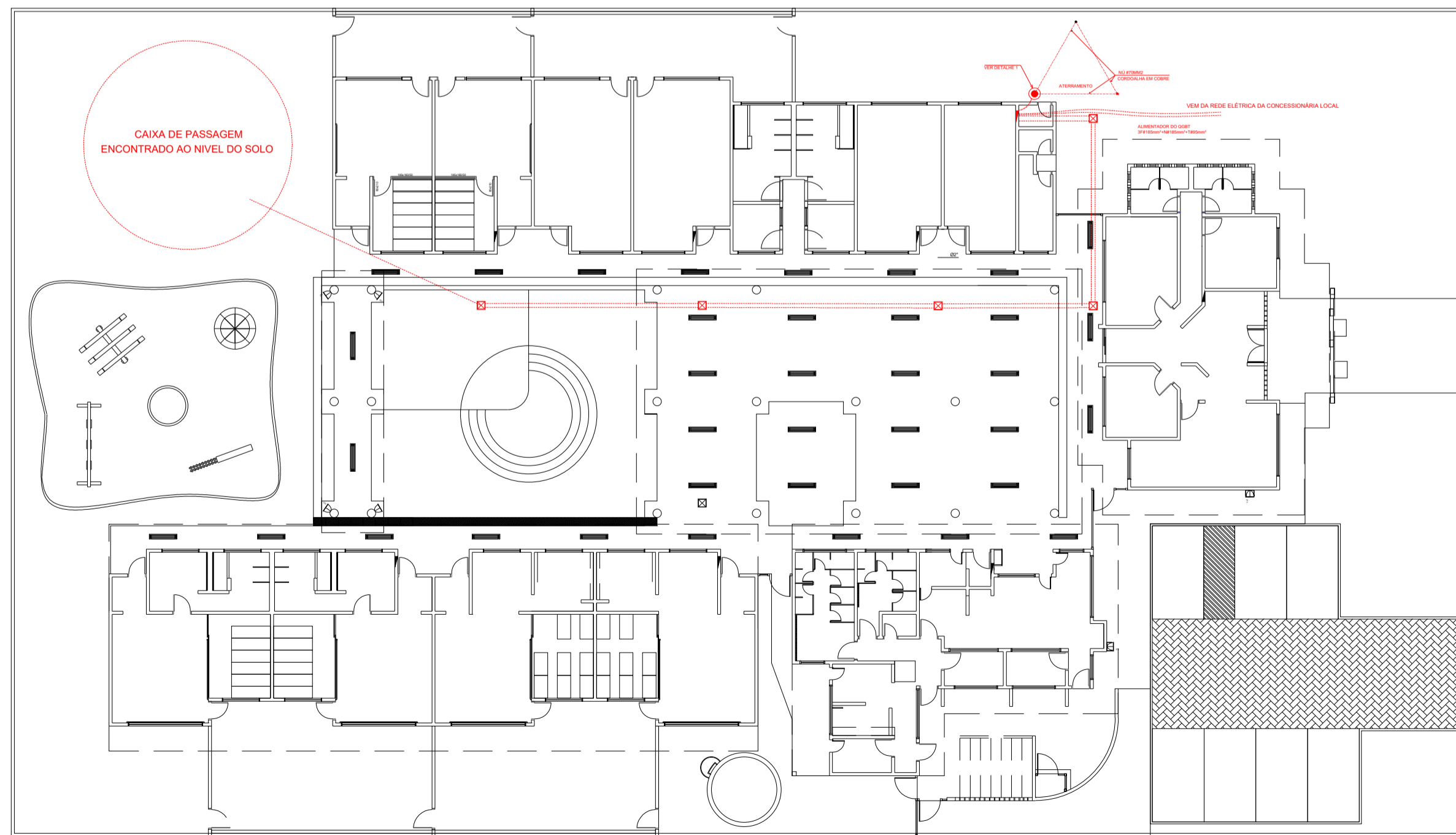
PLANTA BAIXA - DISPOSIÇÃO ELÉTRICA EXISTENTE
