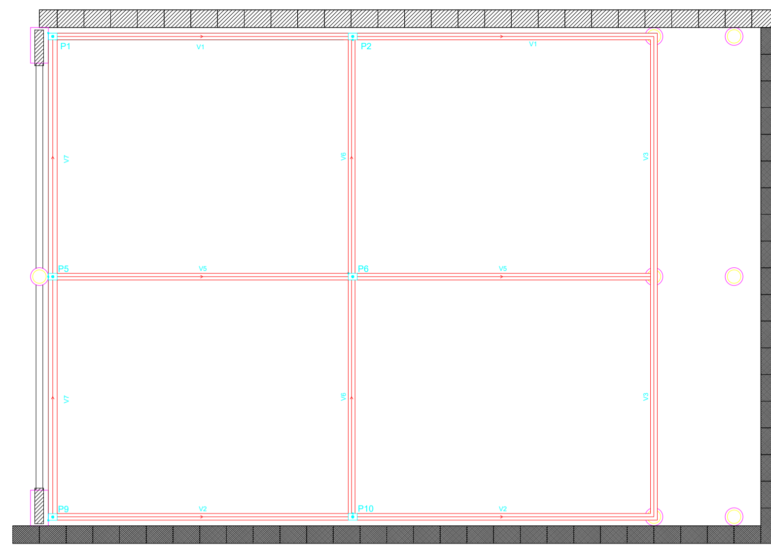
Vigas Cinto
