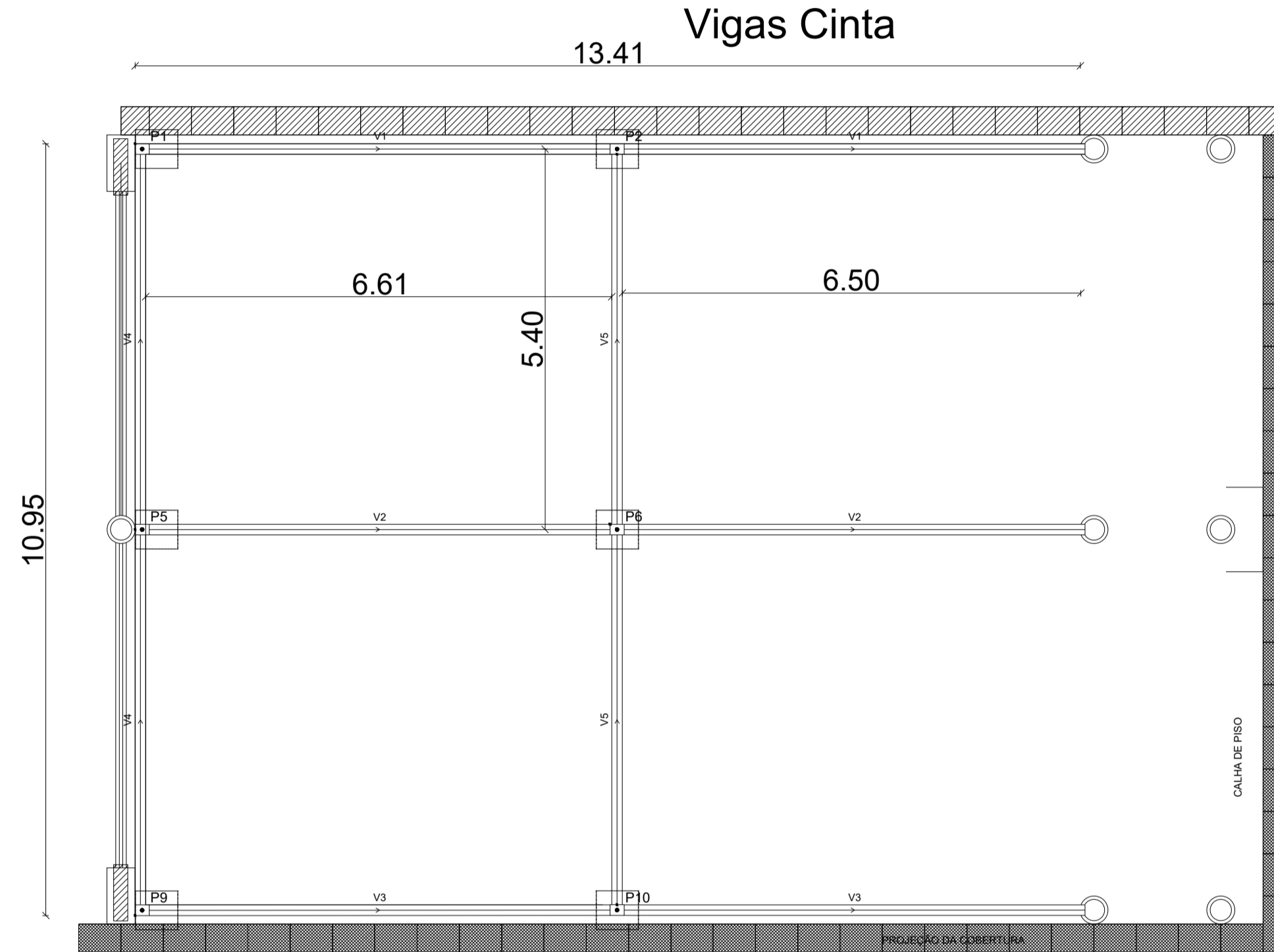
Cotas
