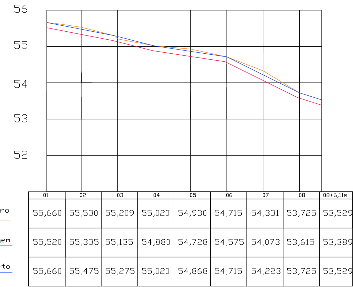
Perfil Longitudinal Dário Souza ESCALA Hor: 1/500 ESCALA Ver: 1/50
