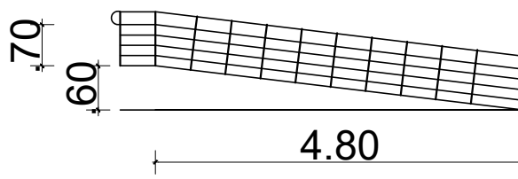
CORTE C-D
