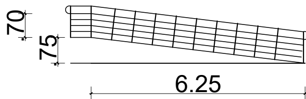
CORTE A-B
