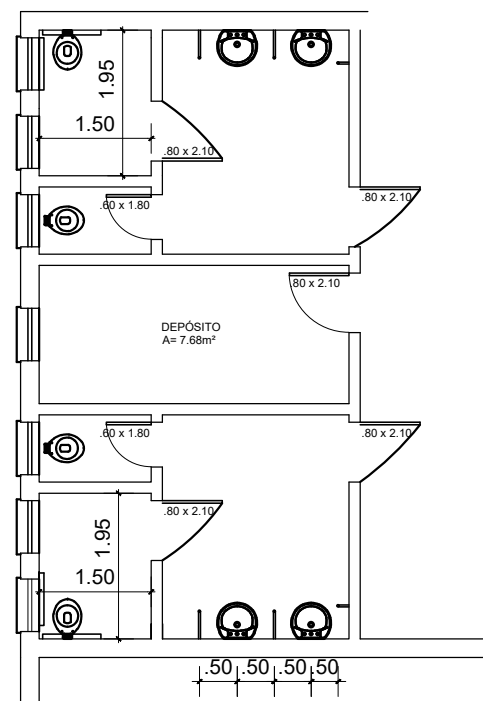
Situação Final
