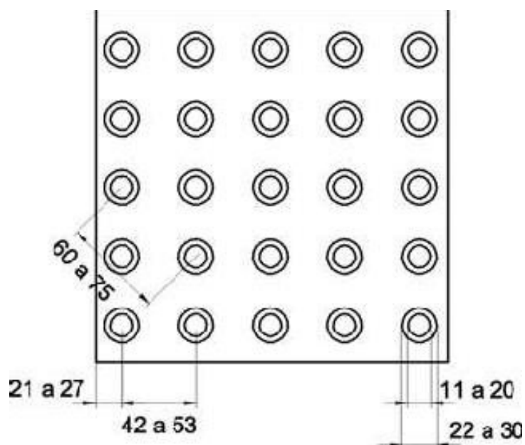
Imagem 06: Ladrilho Hidráulico Alerta – VERMELHO
