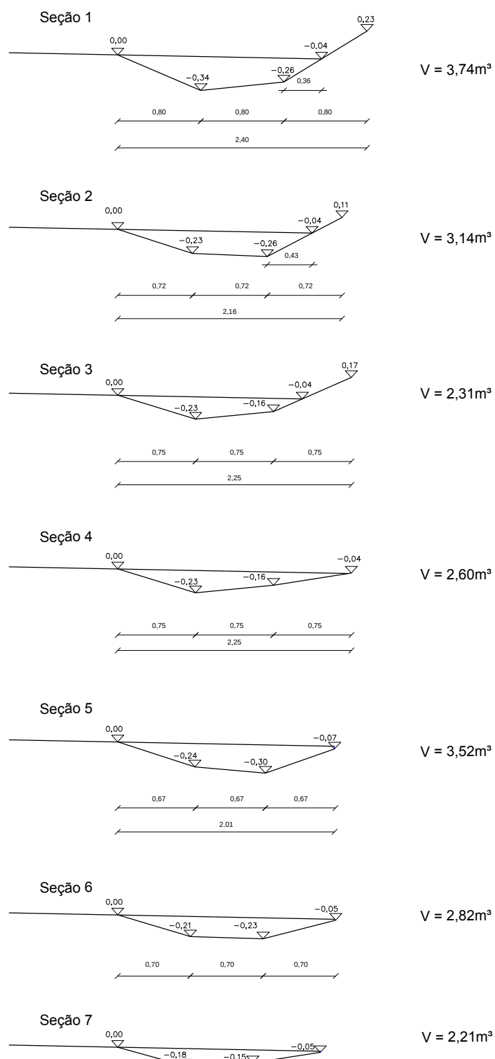
Seções transversais da vala ESCALA: 1/50
